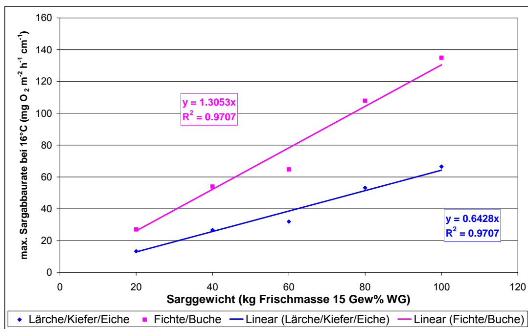
Abb. 3: Abhängigkeit der Abbaurrate eines Leichnams in Abhängigkeit vom Gewicht des Leichnams (EIGENE DARSTELLUNG)
