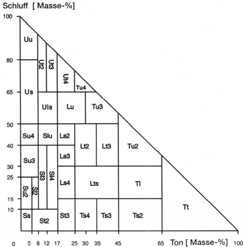
Abbildung 1: Bodenartendiagramm der Bodenartenuntergruppen des Feinbodens (nach KA5, 2005)
