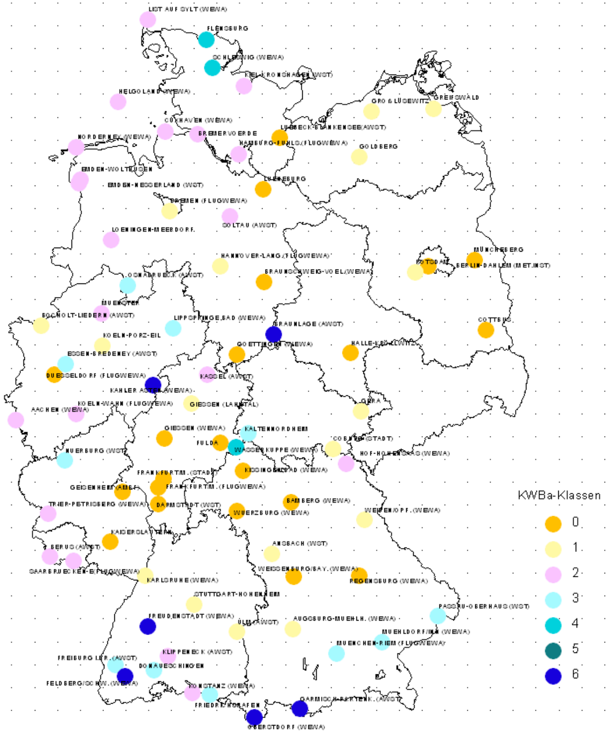
Abb. 1: Klimatische Wasserbilanz an 80 Standorten in Deutschland (EIGENE DARSTELLUNG)
