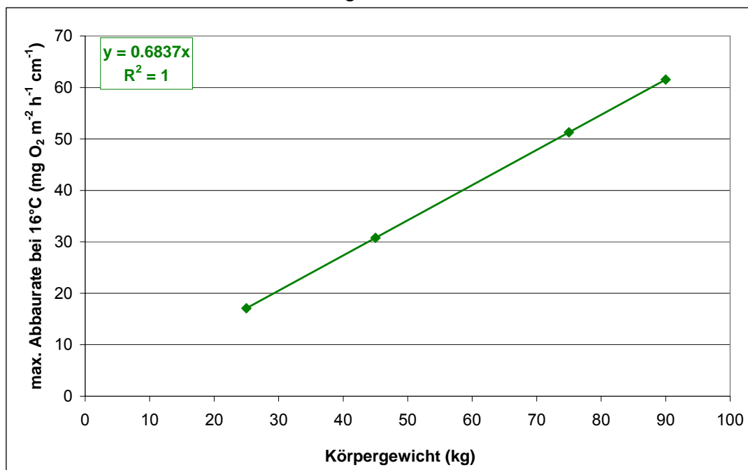
Abb. 2: Abhängigkeit der Abbaurate eines Leichnams in Abhängigkeit vom Gewicht des Leichnams (EIGENE DARSTELLUNG)
